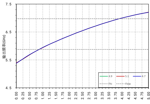
RFOUT输出频率 VS VCC
